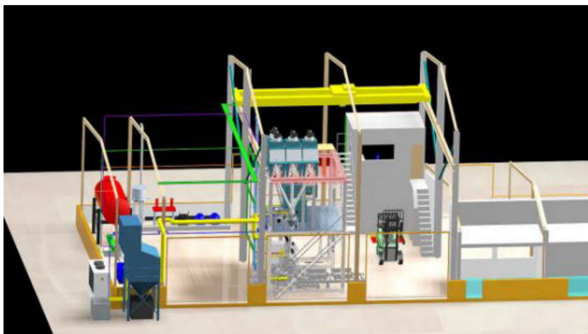
Esquema de la planta de estabilización de mercurio de Mayasa. / LT
